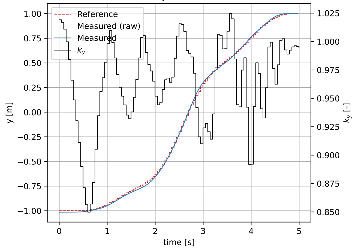
y State
